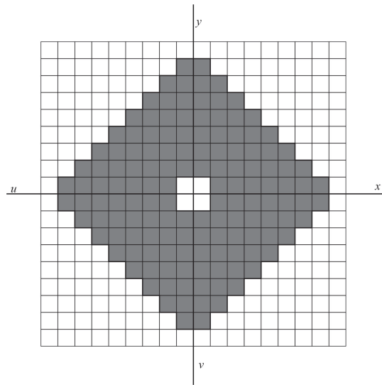
Slika 3.2: Region S_8
